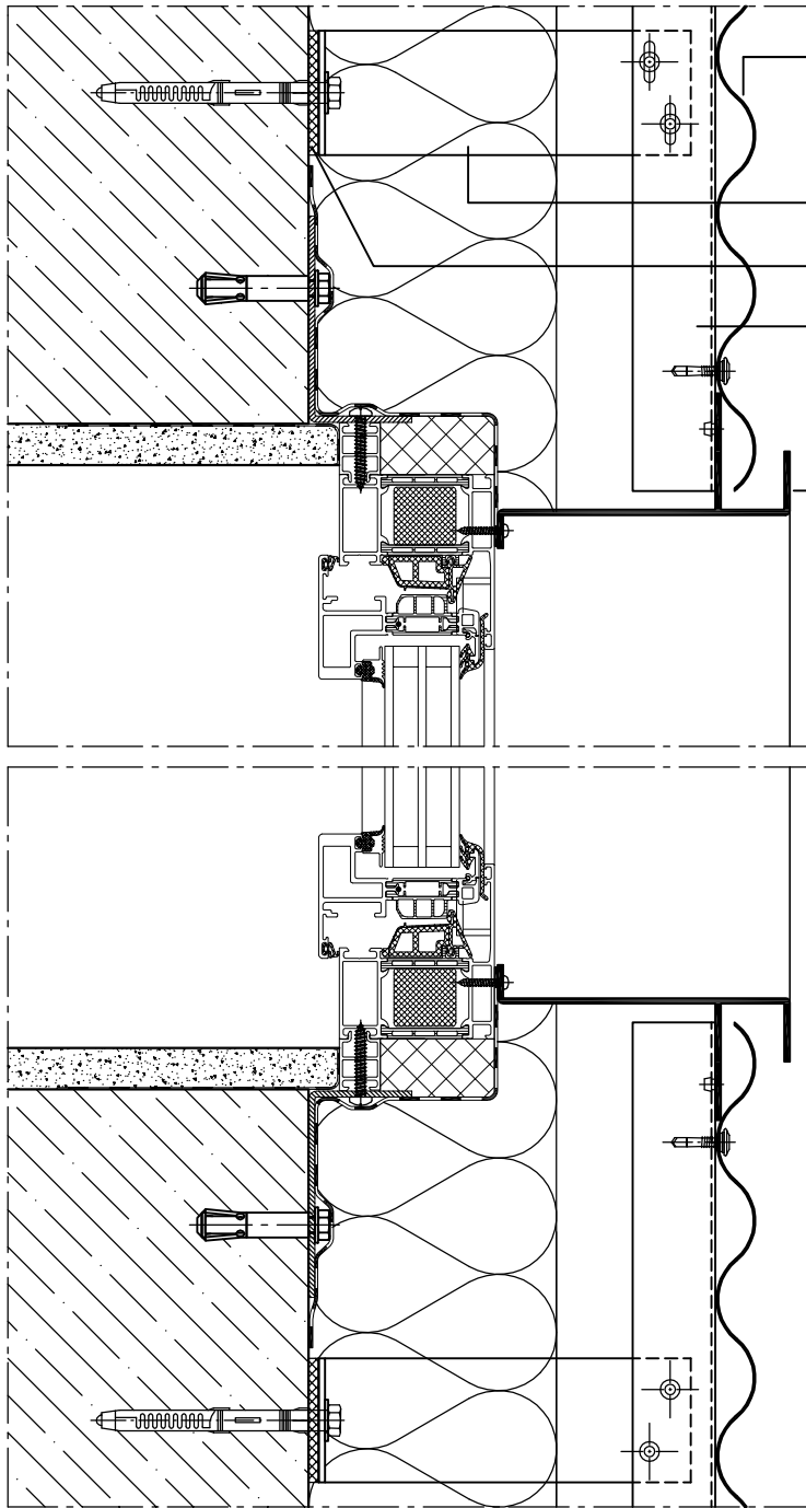
Vertikalschnitt
